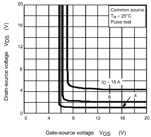
Fig. 8.4 V_{DS} - V_{GS}
